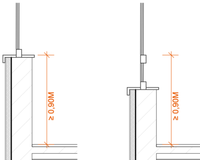
Figure 16 : Hauteurs des allèges de fenêtres
