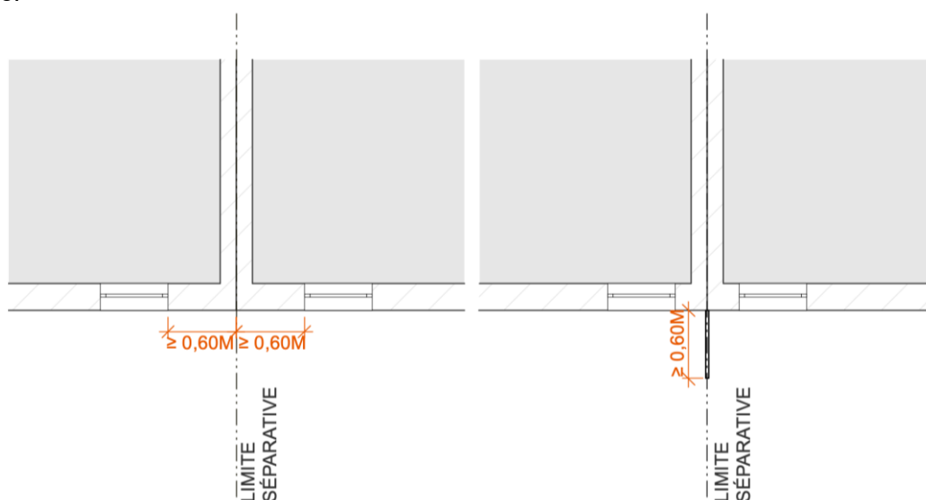
Figure 12 : Distance entre ouvertures
