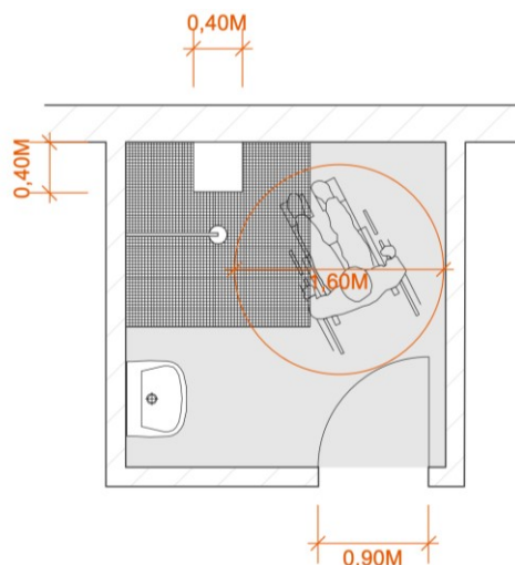
Figure 23 : Cabine de douche
