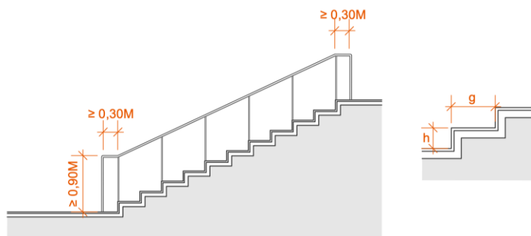
Figure 20 : Escaliers et mains courantes
