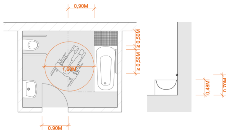
Figure 22 : Salle de bains
